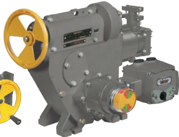
МЭОФ...02К с блоком КИМ1
