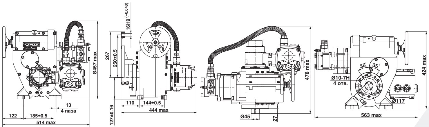
Рычажное исполнение (МЭО)
