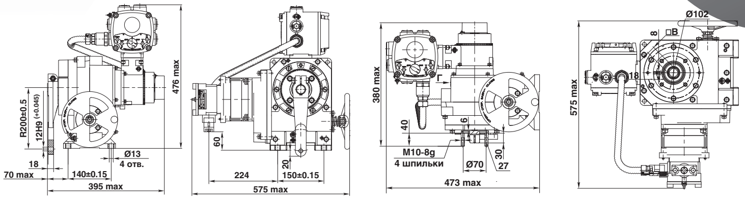
Рычажное исполнение (МЭО)
